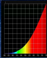
Spektrum světla ohně (spektrum noci)
