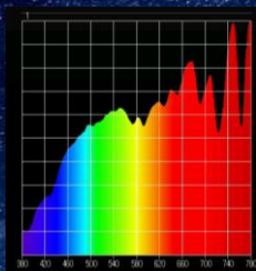
Spektrum podvečerního světla
