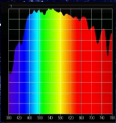
Spektrum denního světla
